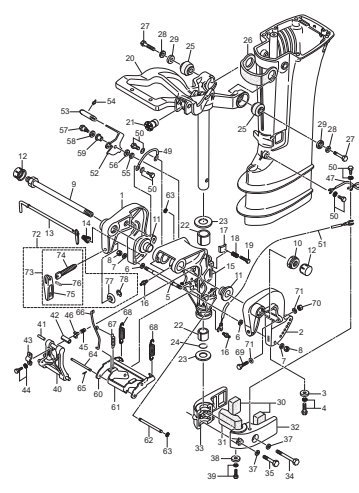
Fig. 10 BRACKET ブラケット
