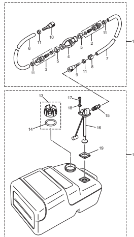
Fig.16 FUEL TANK フエルトンク
