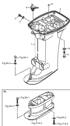
Fig. 8 DRIVE SHAFT HOUSING ドライブシャフトハウジング
