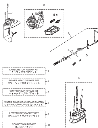
Fig.21 ASSEMBLY · KIT PARTS アッセンブリ・キットパーツ
