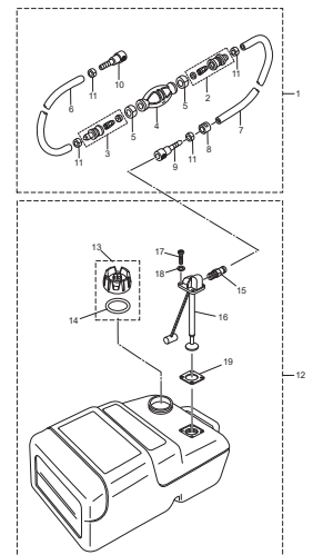
Fig.17 FUEL TANK フエルトンク
