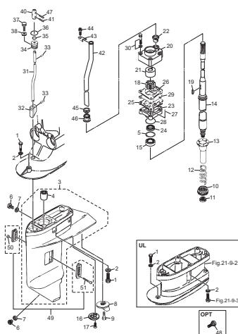
Fig. 9A GEAR CASE (DRIVE SHAFT) ギヤケース (ドライブシャフト)
