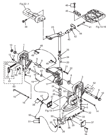
Fig. 23 BOTTOM COWL · SHIFT ボトムカウル・シフト
