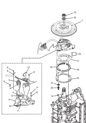
Fig. 8 MAGNETO マグネット
