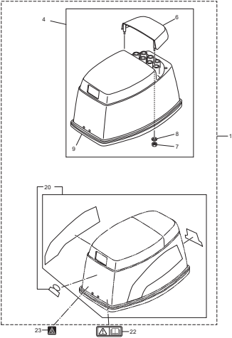
Fig. 32 OPTIONAL PARTS (5) オプションパーツ (5)
