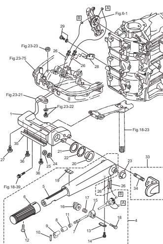
Fig. 22 TILLER HANDLE (F TYPE) ティラハンドル (Fタイプ)
