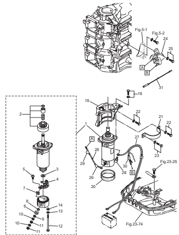
Fig. 9 ELECTRIC PARTS (STARTER MOTOR) エレクトリックパーツ (スタータモータ)
