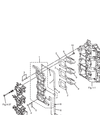
Fig. 3 INTAKE MANIFOLD · REED VALVE インテークマニホールド・リードバルブ
