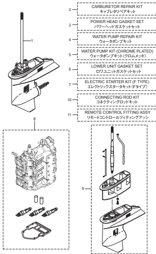
Fig. 33 ASSEMBLY KIT PARTS アッセンブリ・キットパーツ
