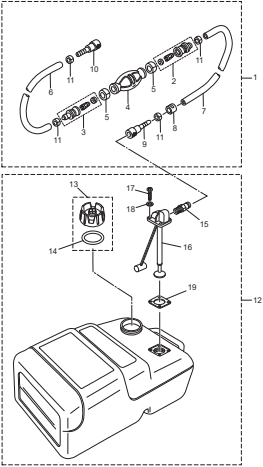
Fig. 33 ASSEMBLY KIT PARTS アッセンブリ・キットパーツ
