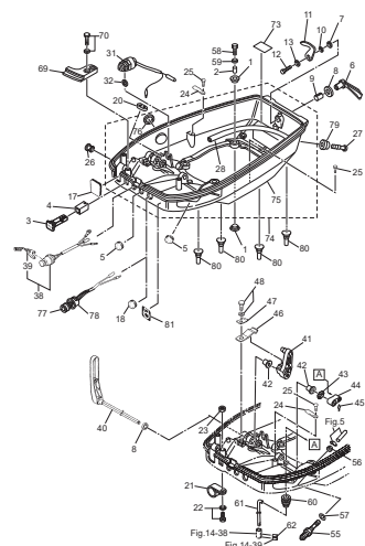
Fig. 23 BOTTOM COWL · SHIFT ボトムカウル・シフト
