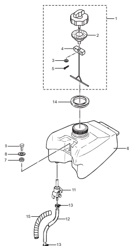
Fig. 11 FUEL TANK フュエルタンク
