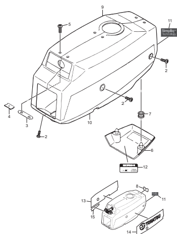
Fig. 13 ASSEMBLY • KIT PARTS アセンブリ・キットパーツ
