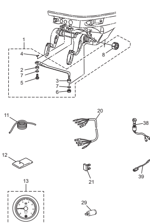
Fig. 28 ACCESSORIES (1) アクセサリ (1)
