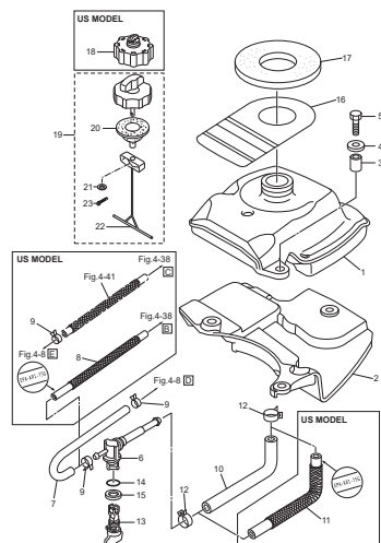
Fig. 15 FUEL TANK フュエルタンク
