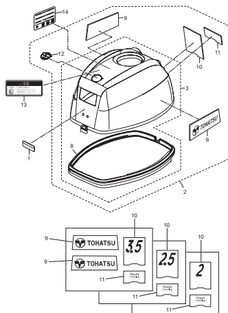
Fig. 17 ASSEMBLY · KIT PARTS アセンブリ・キットパーツ
