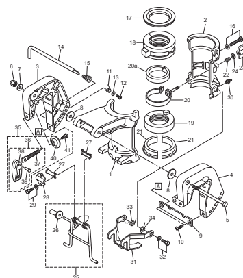
Fig. 9 BRACKET · REVERSE LOCK ブラケット · リバースロック
