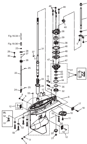
Fig.11 GEAR CASE (DRIVE SHAFT) ギヤケース (ドライブシャフト)
