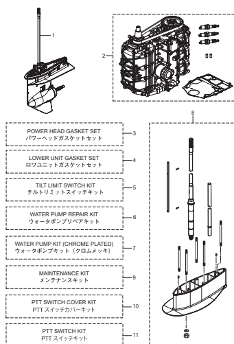
Fig. 26 ASSEMBLY · KIT PARTS アッセンブリ・キットパーツ
