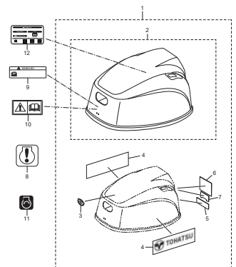
Fig.15 TOP COWL トップカウル
