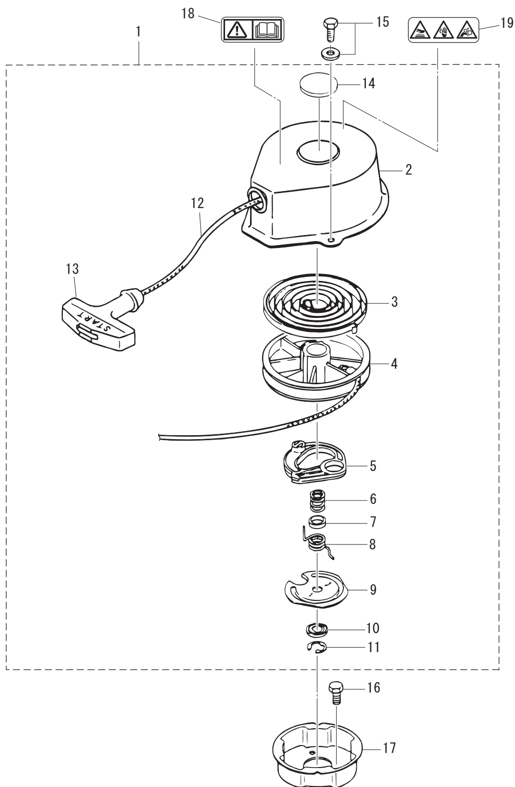
Fig. 4 RECOIL STARTER リコイルスタータ
