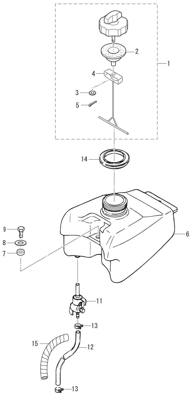
Fig. 11 FUEL TANK フュエルタンク
