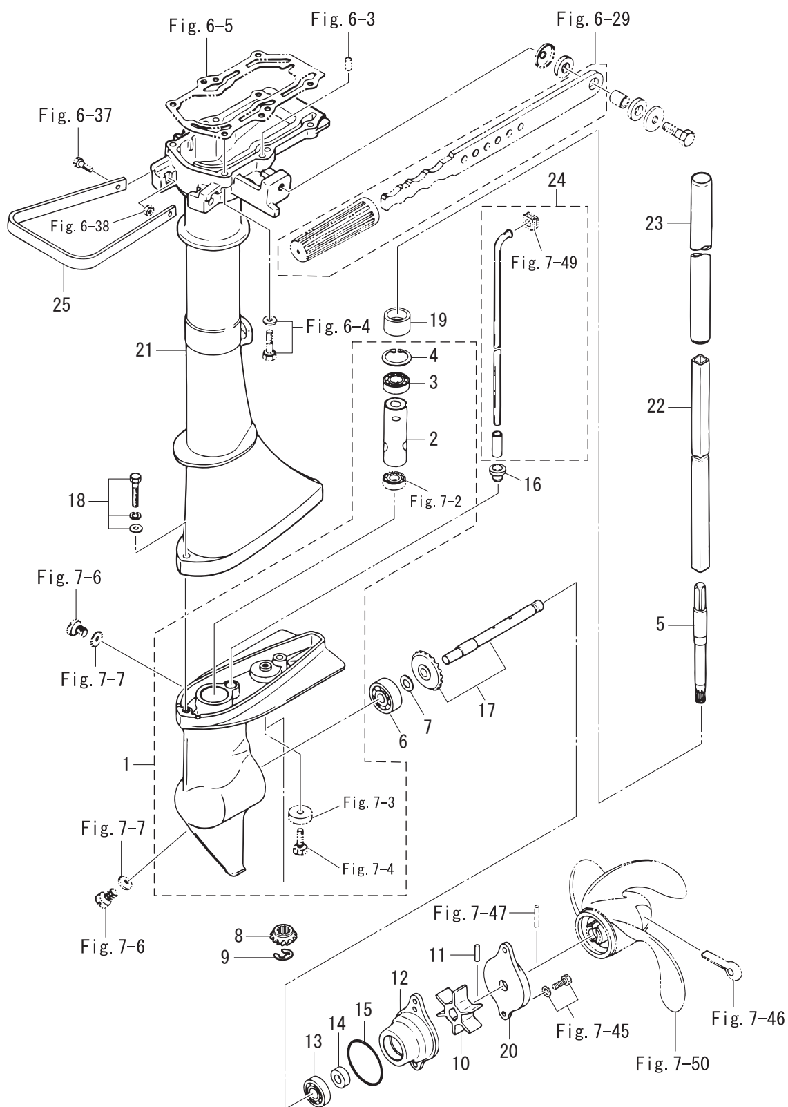
Fig. 8 DRIVE SHAFT HOUSING · GEAR CASE (M3. 5A2) ドライブシャフトハウジング・ギヤケース (M3. 5A2)
