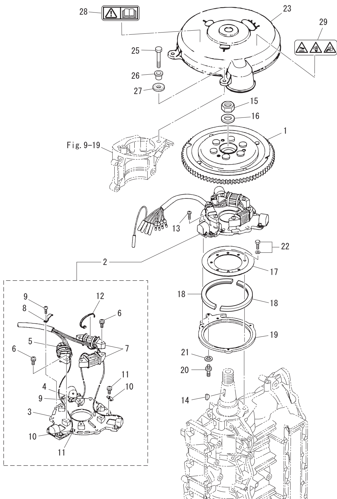
Fig. 8 MAGNETO マグネト
