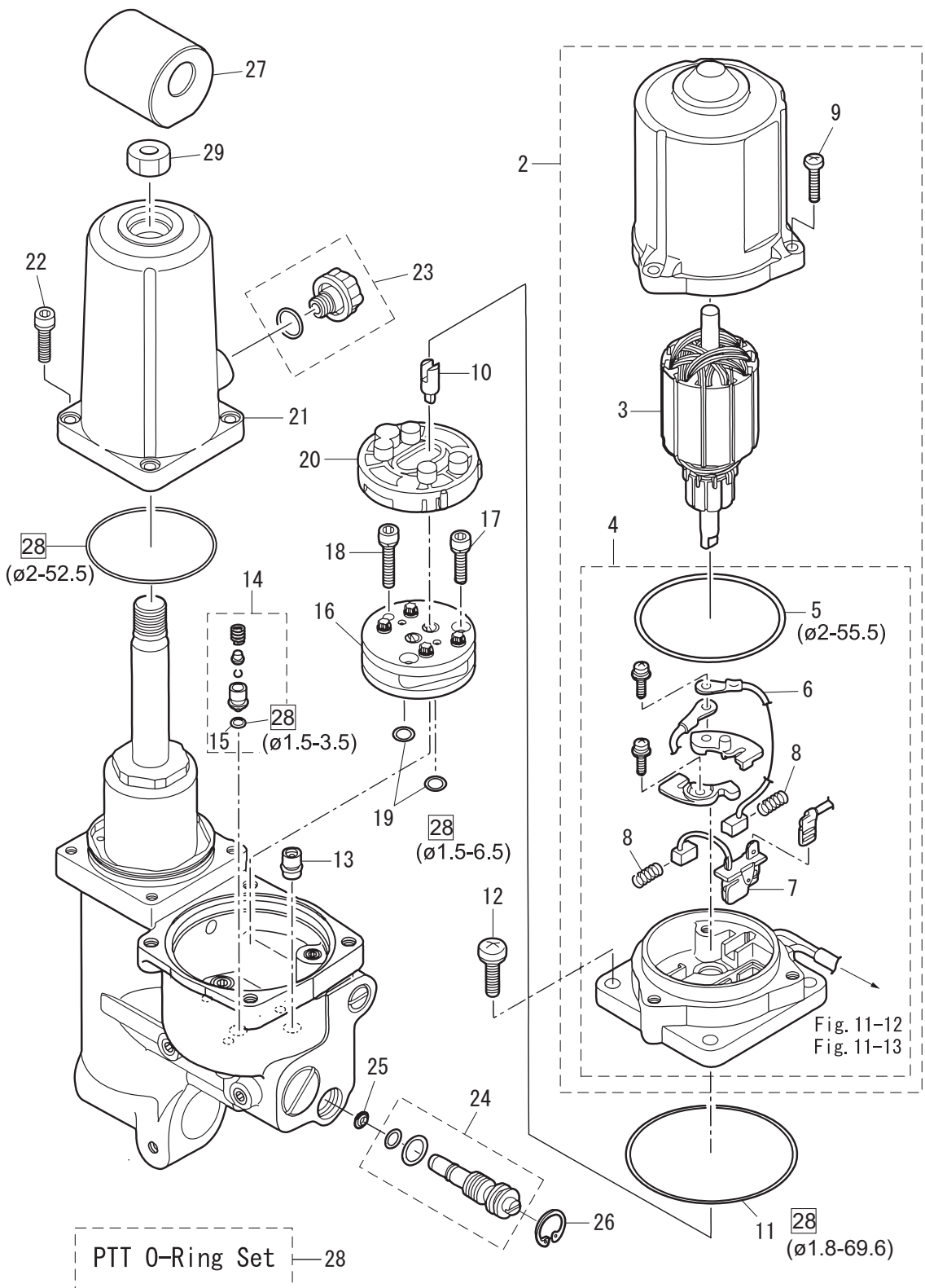
Fig. 21 POWER TRIM&TILT パワートリム&チルト
