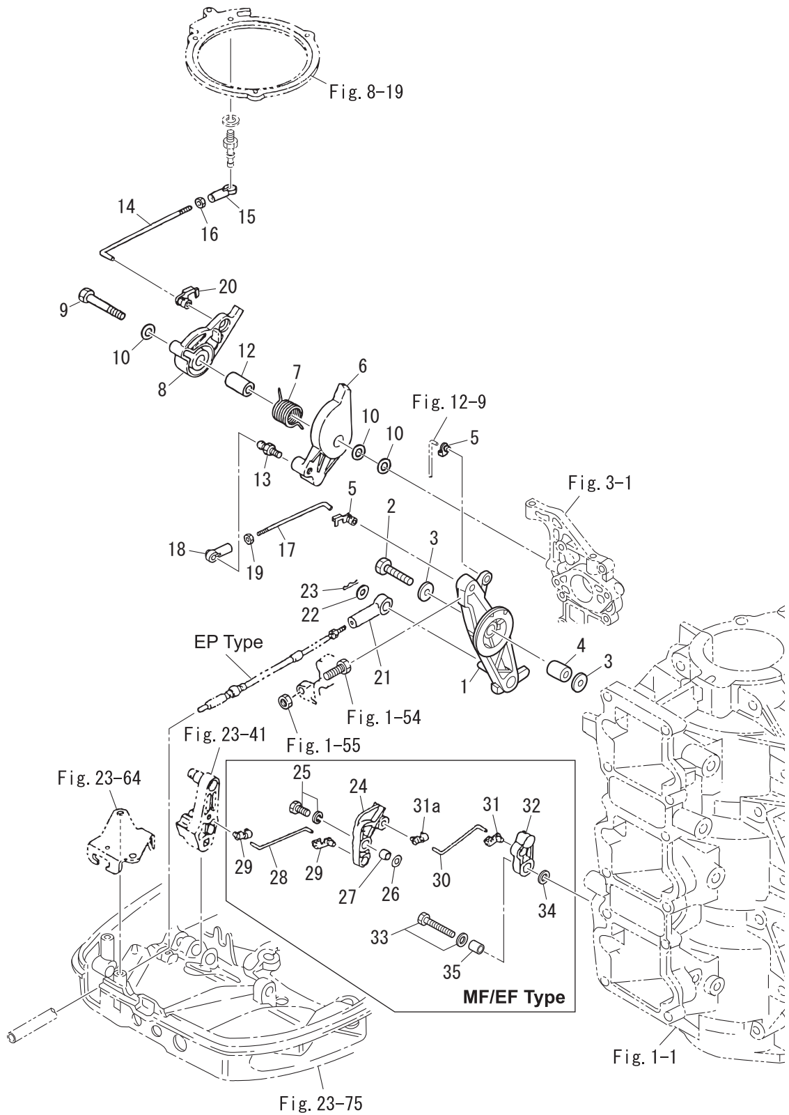
Fig. 6 THROTTLE スロットル
