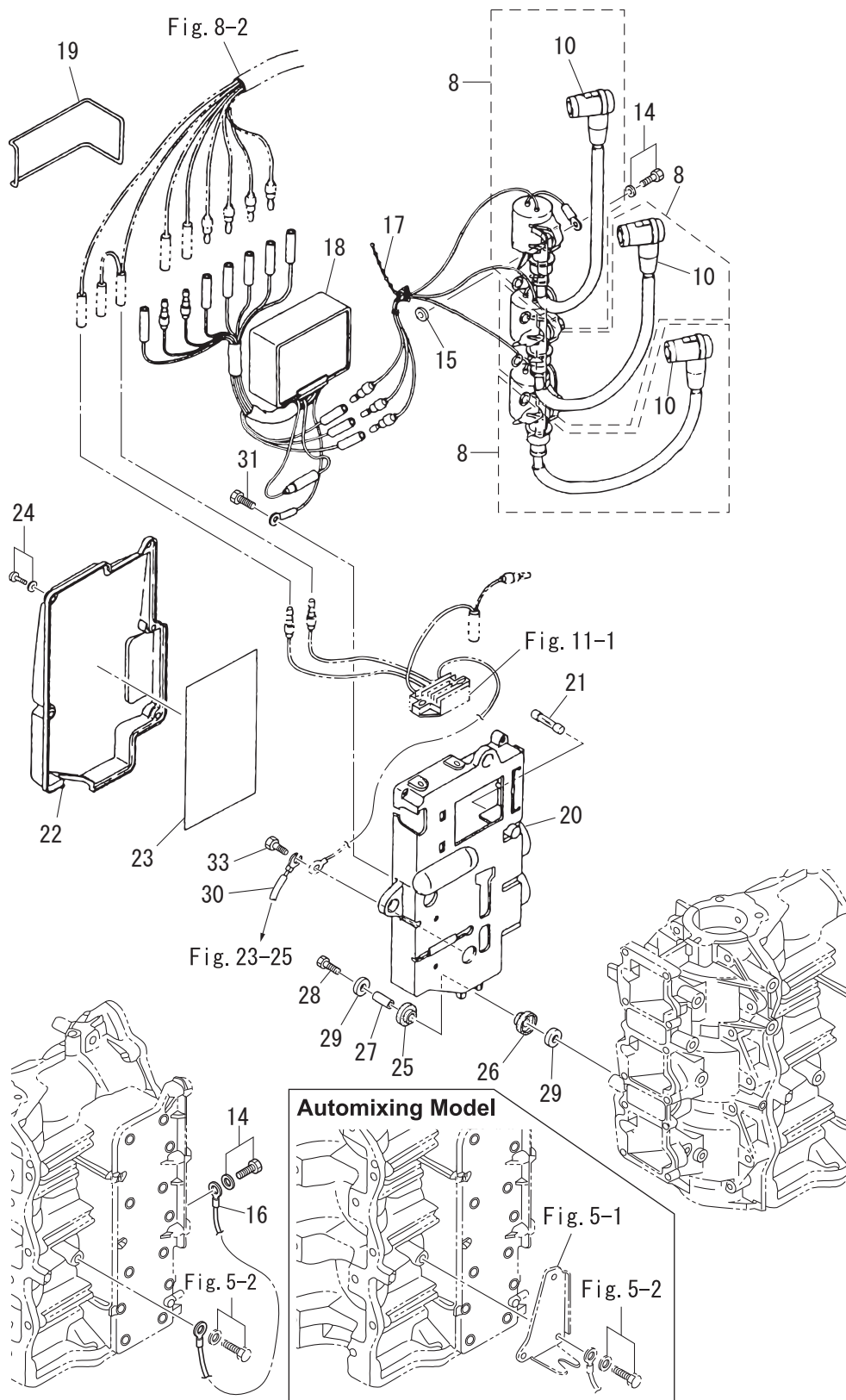
Fig. 10 ELECTRIC PARTS (C. D. UNIT) エレクトリックパーツ (C.D. ユニット)
