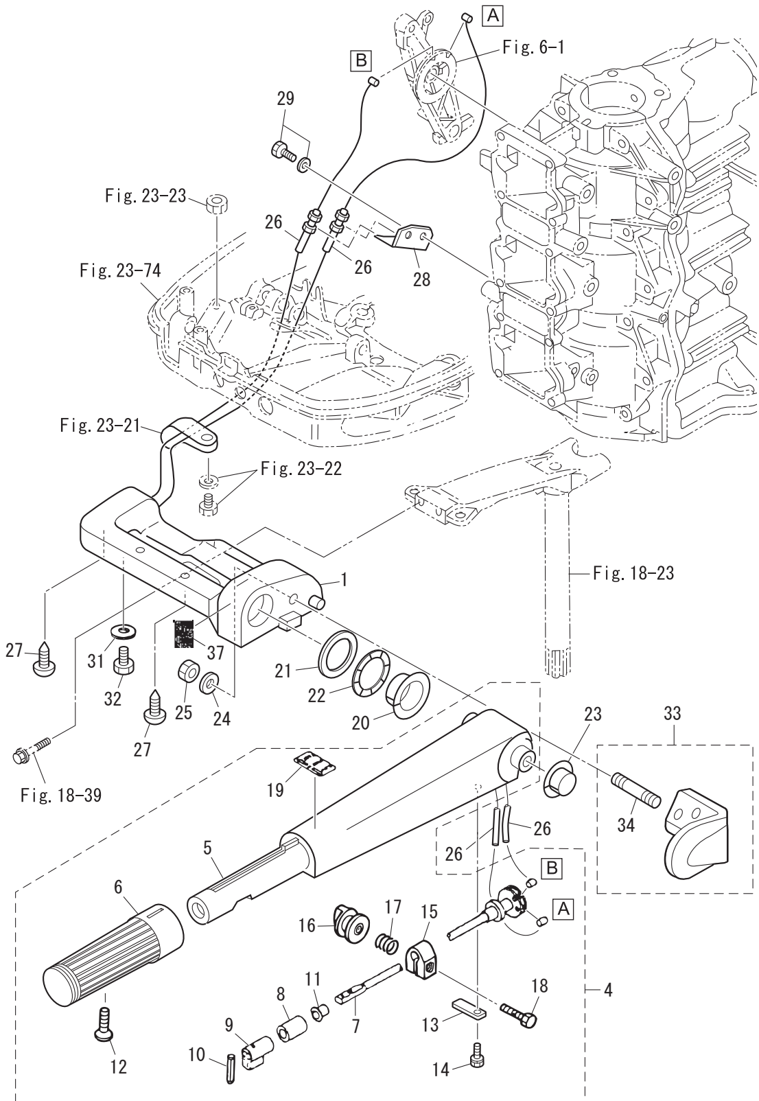
ティラハンドル (Fタイプ)
