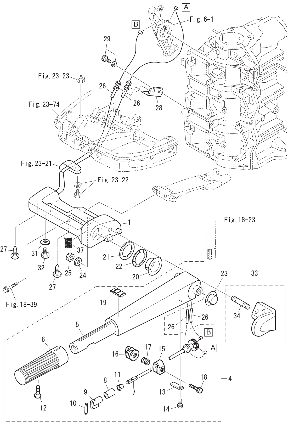
ティラハンドル (Fタイプ)
