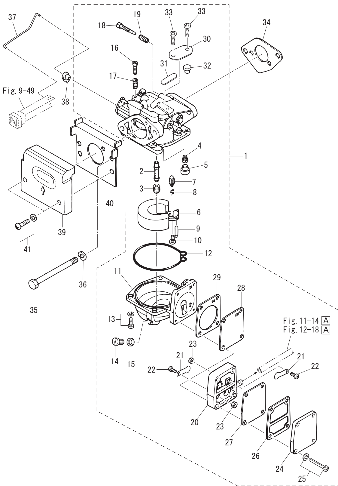
CARBURETOR キャブレタ
