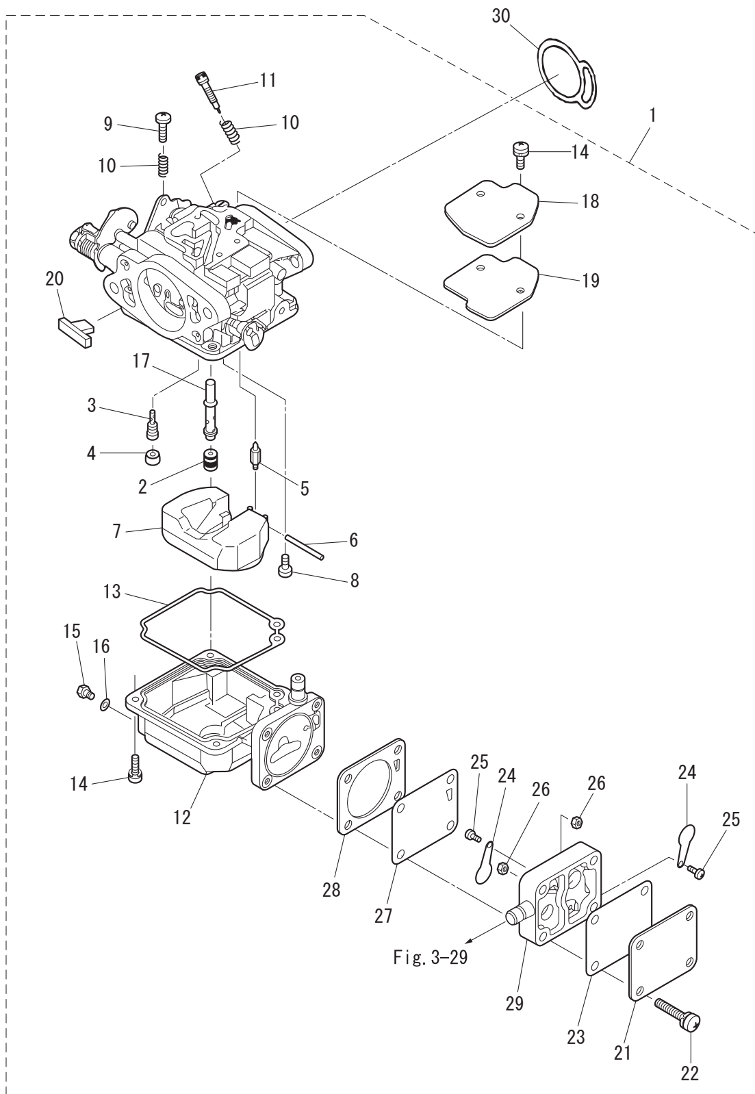
Fig. 4 CARBURETOR キャブレタ
