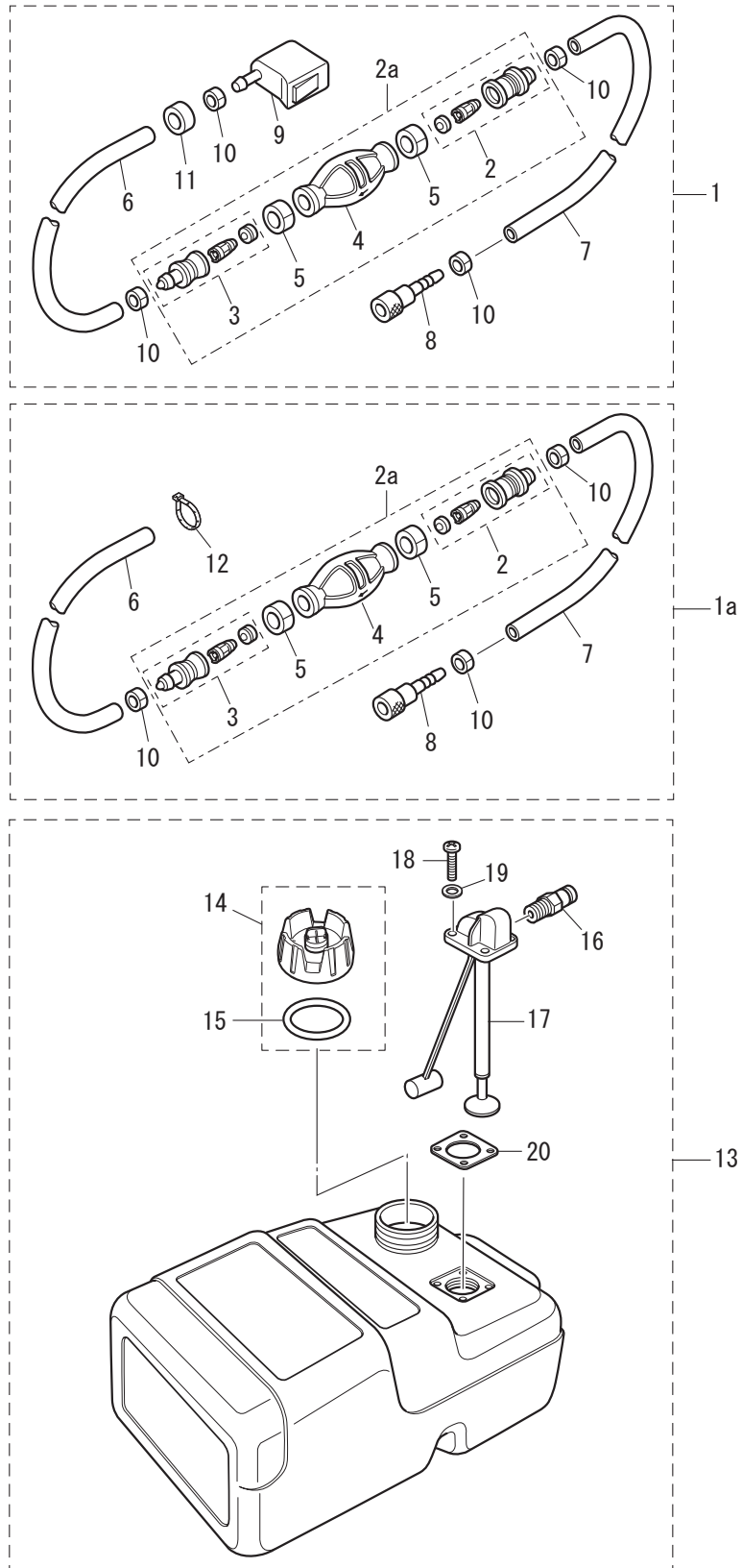
Fig. 21 FUEL TANK フュエルタンク
