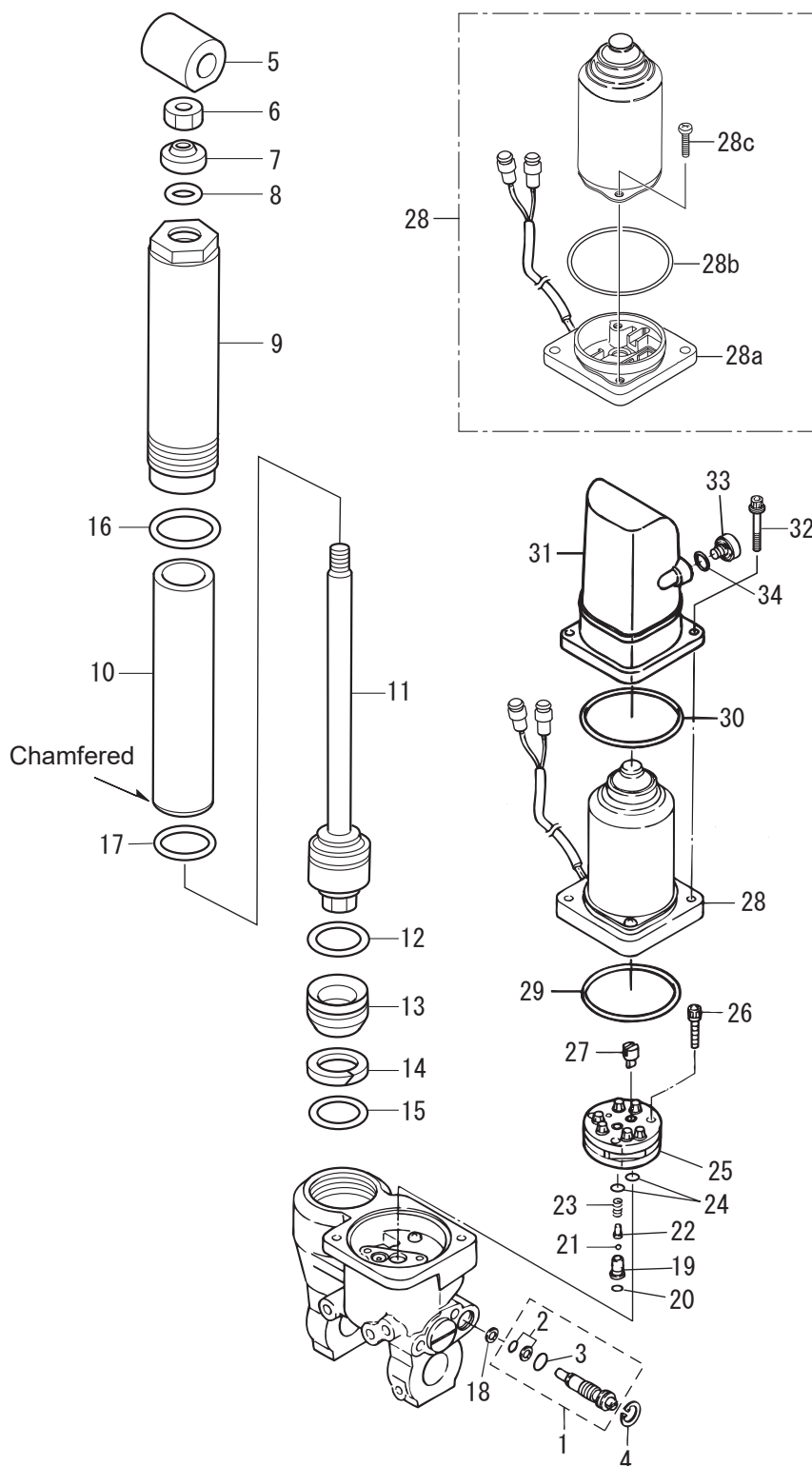
Fig. 15 POWER TILT パワーチルト
