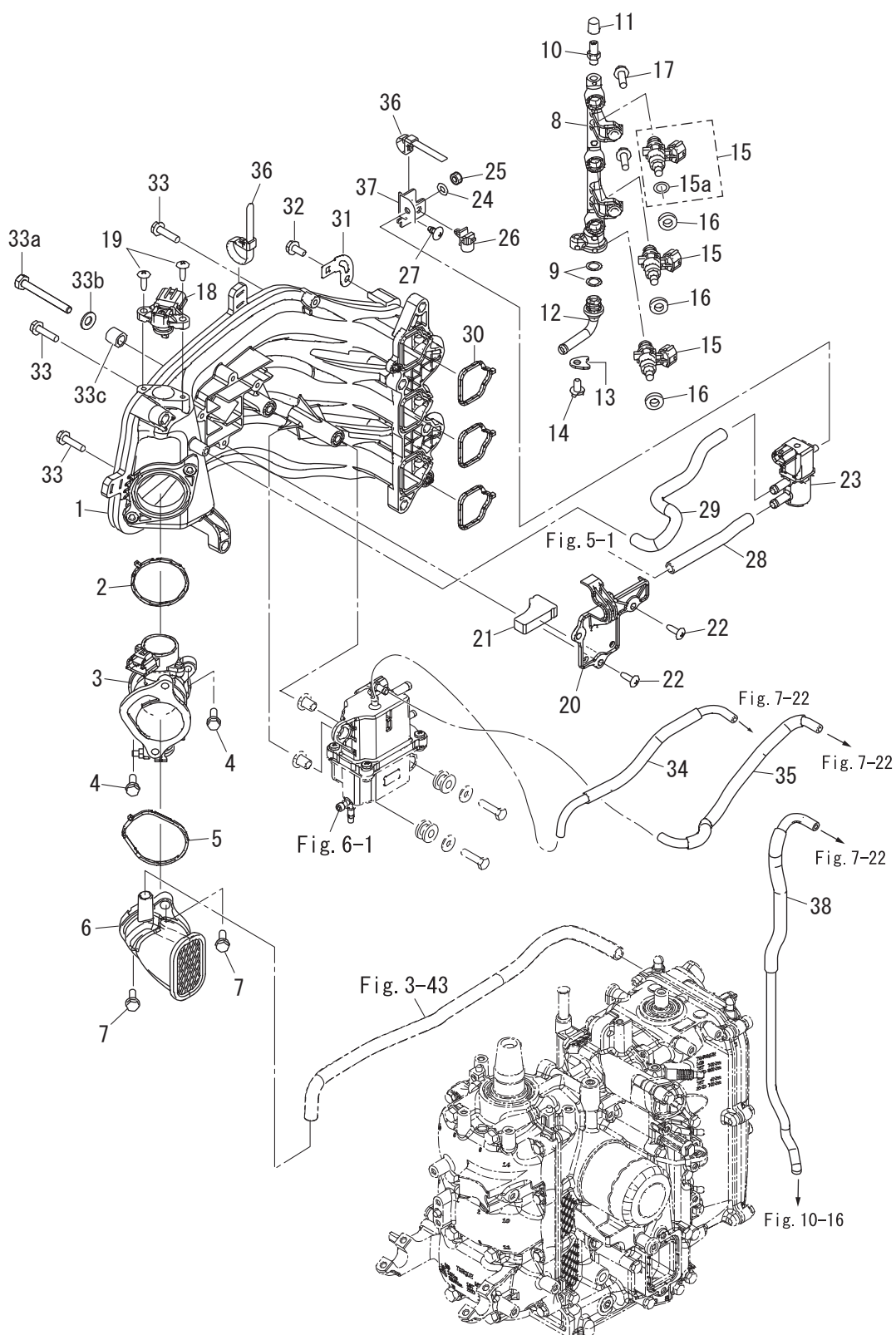
Fig. 5 INTAKE MANIFOLD インテークマニホールド
