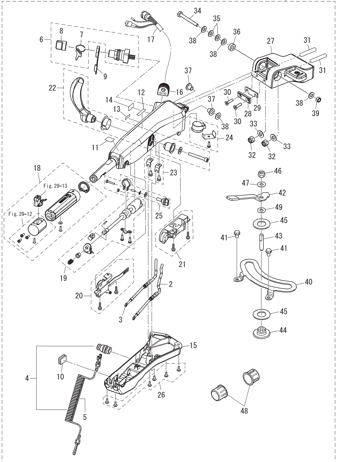
Fig. 23 MULTI TILLER HANDLE マルチティラハンドル
