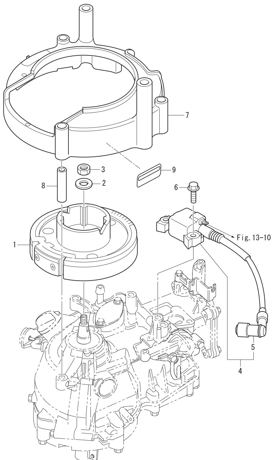
Fig. 7 MAGNETO マグネト
