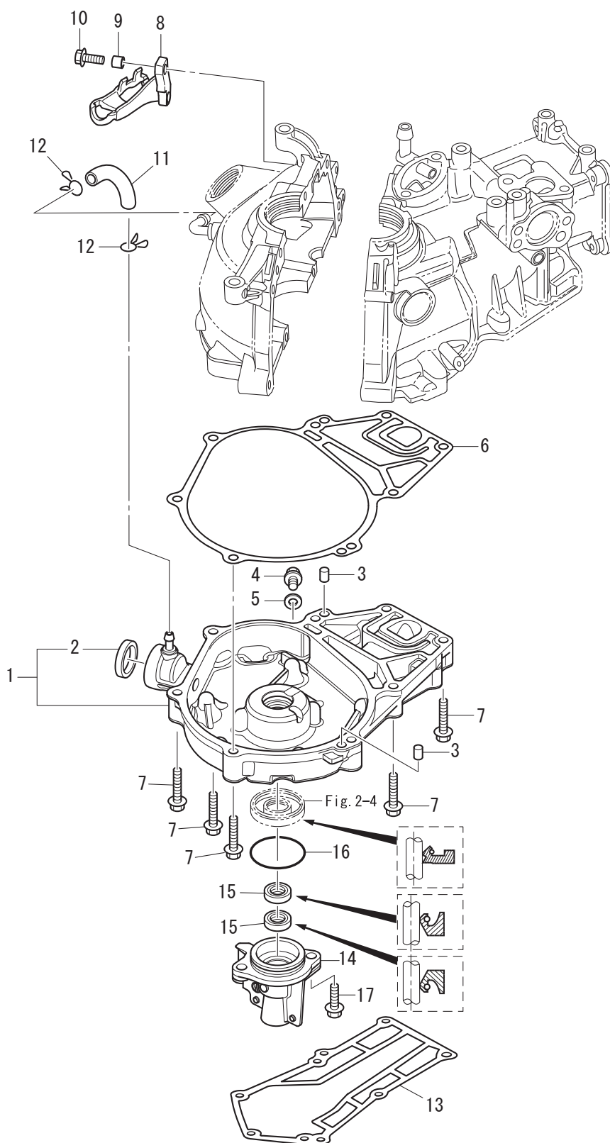
Fig. 3 OIL PAN オイルパン
