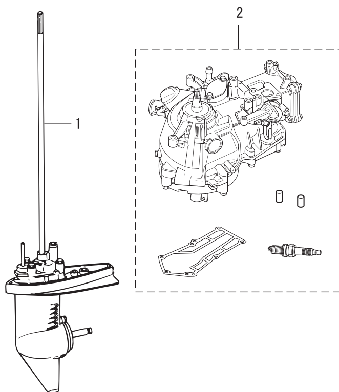
Fig. 17 ASSEMBLY · KIT PARTS アッセンブリ・キットパーツ
