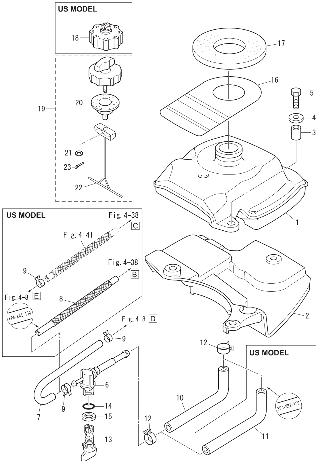
FUEL TANK フュエルタンク
