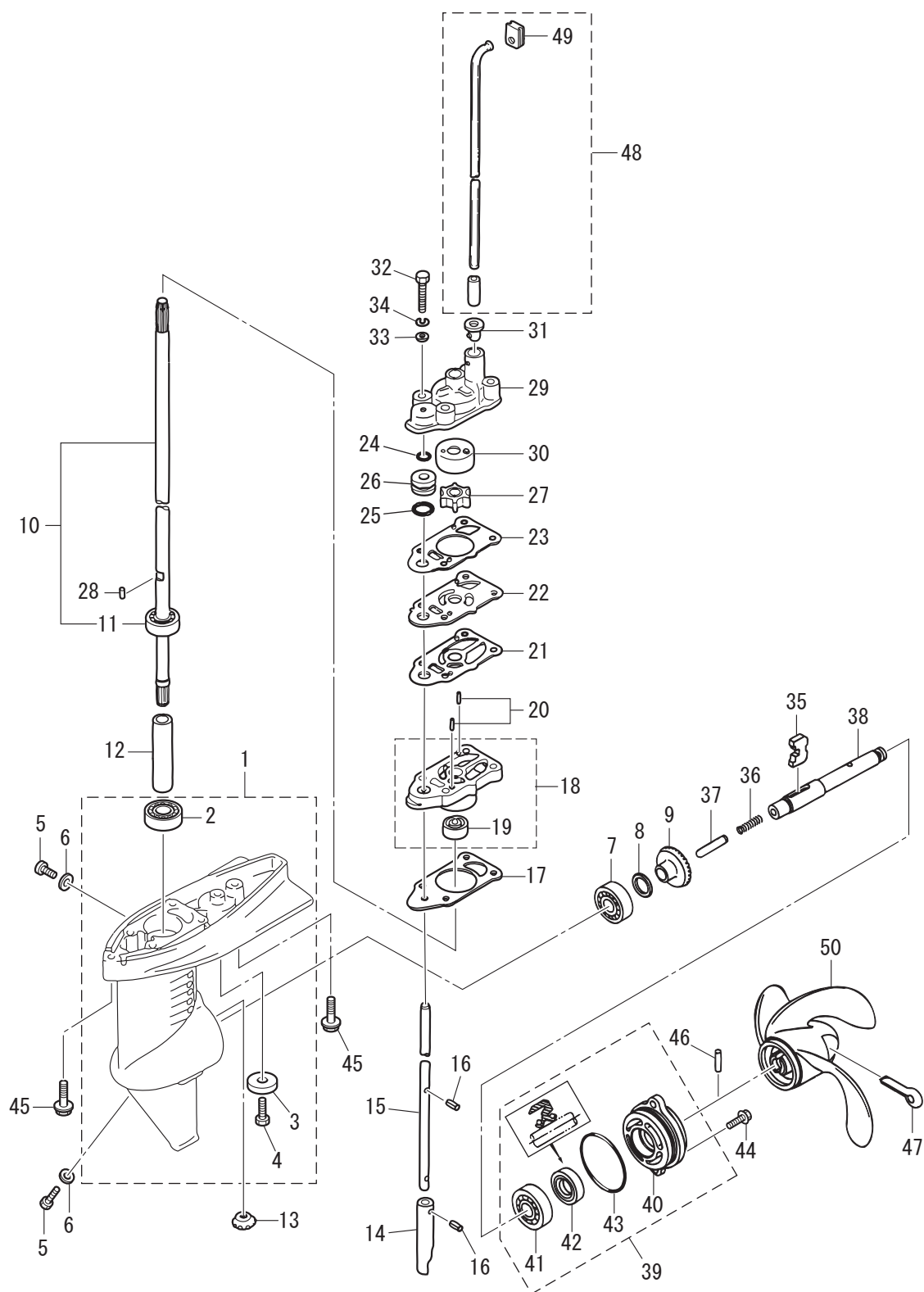
Fig. 10 GEAR CASE ギヤケース
