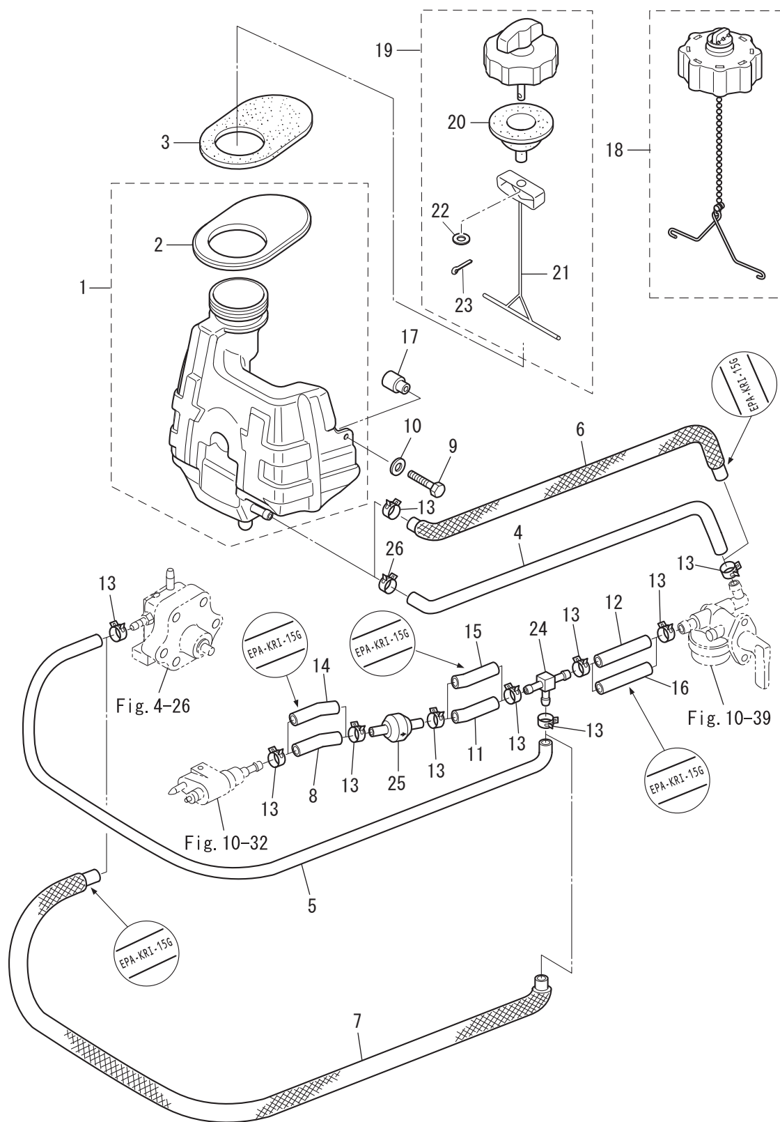
INTEGRAL FUEL TANK インテグラルフュエルタンク
