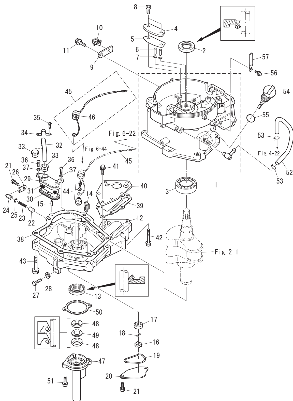
Fig. 1 CYLINDER · OIL PAN シリンダ · オイルパン
