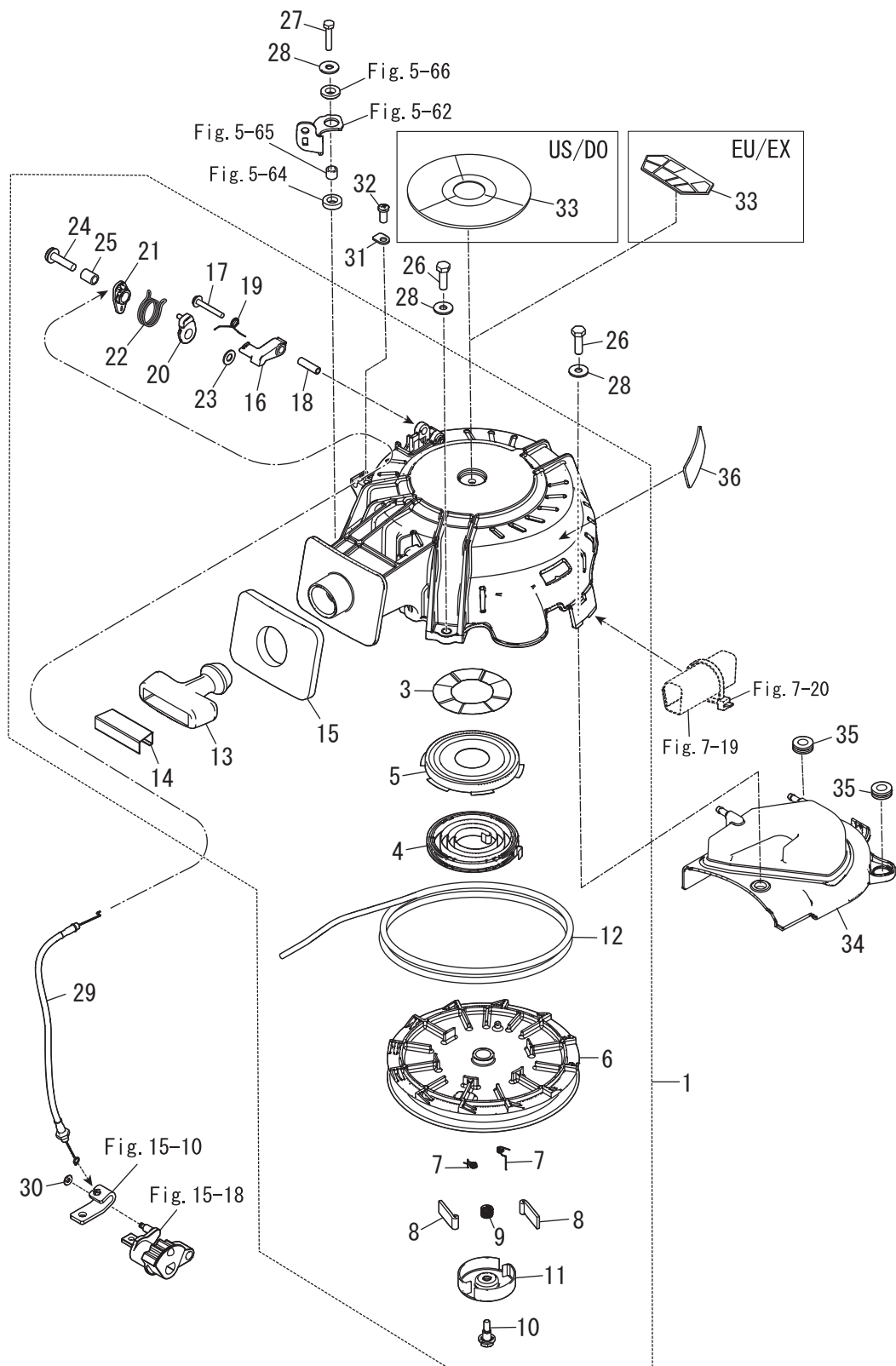
Fig. 6 RECOIL STARTER リコイルスタータ
