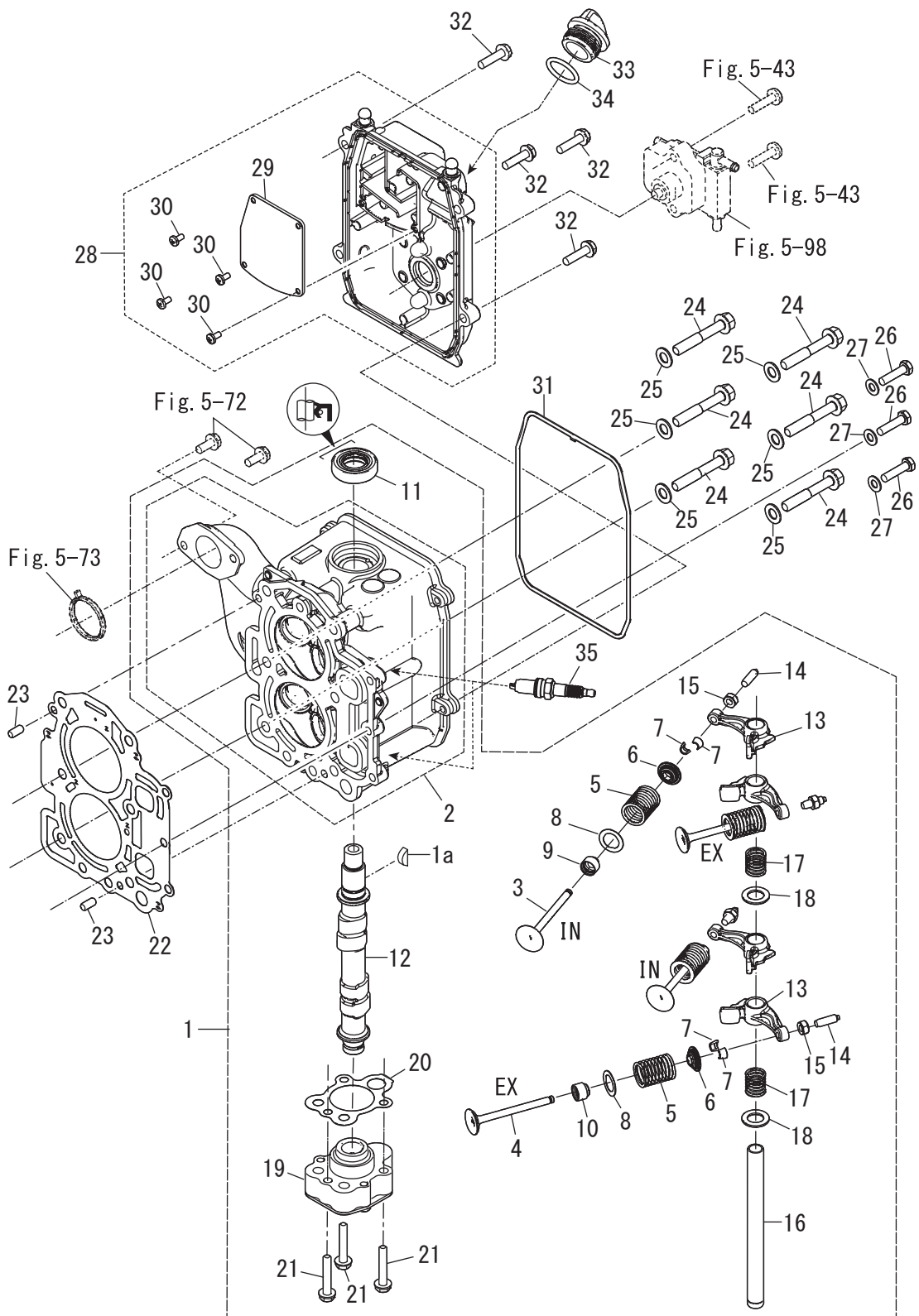
Fig. 3 CYLINDER HEAD · OIL PUMP シリンダヘッド・オイルポンプ
