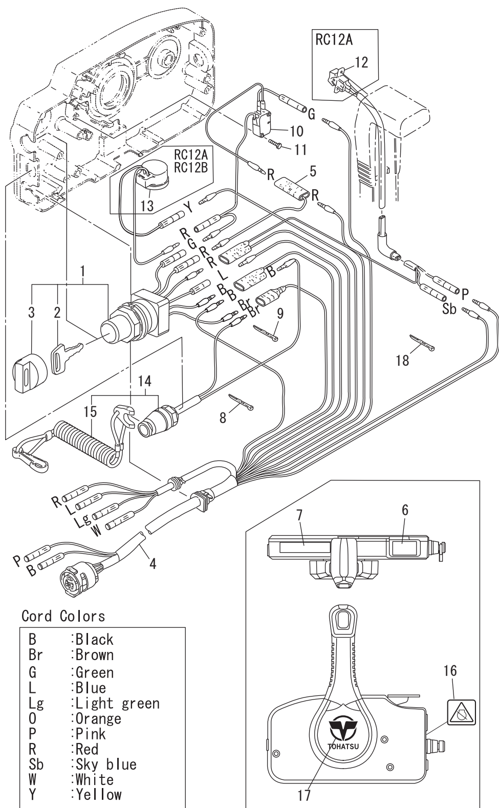
Fig. 19 COMPONENT PARTS OF REMOTE CONTROL (ELECTRIC PARTS) リモコンボックス構成部品(電装品関係)
