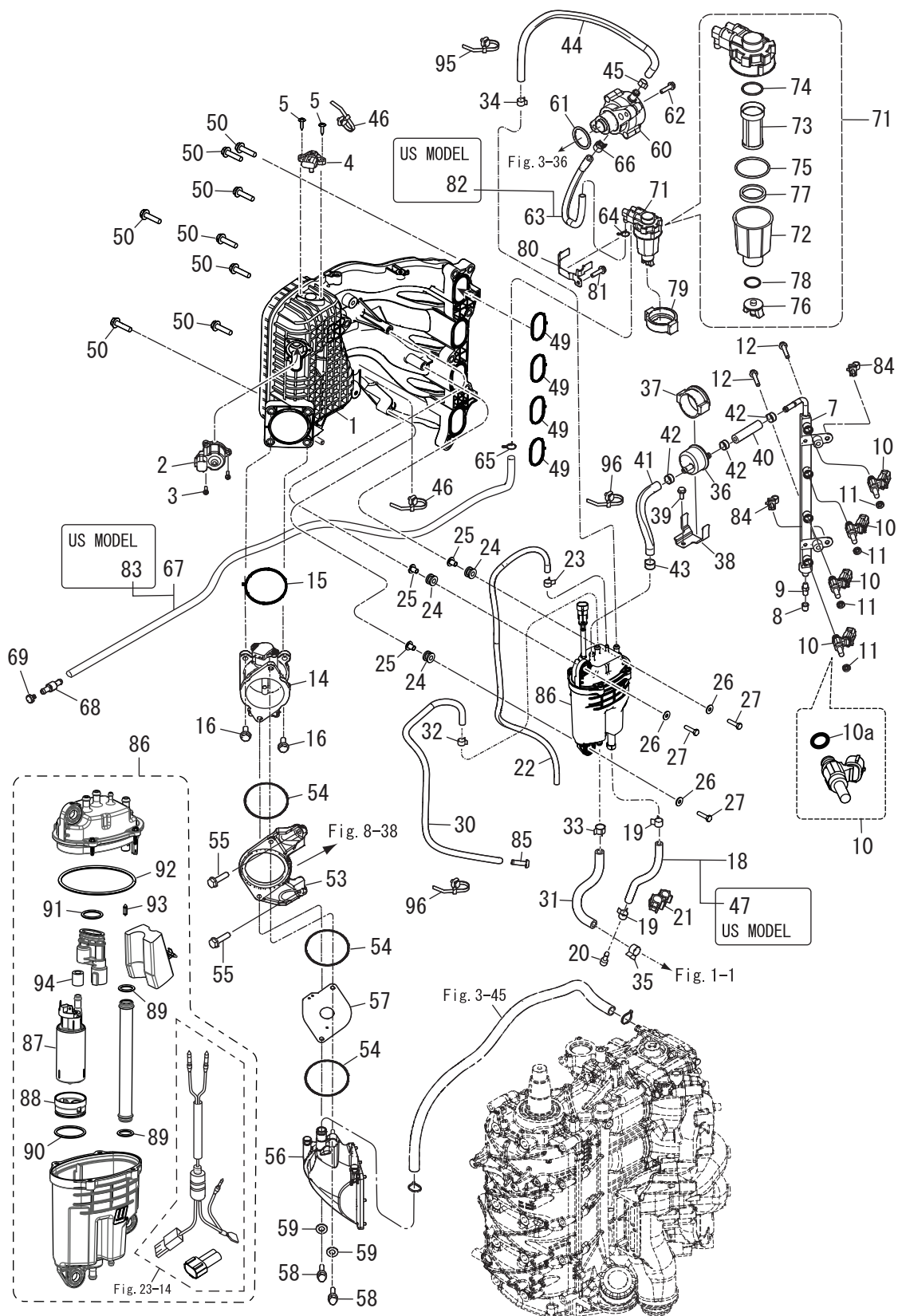
Fig. 5 INTAKE MANIFOLD · FUEL SYSTEM インテークマニホールド · フュエルシステム
