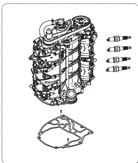
POWER HEAD GASKET SET パワーヘッドガスケットセット
