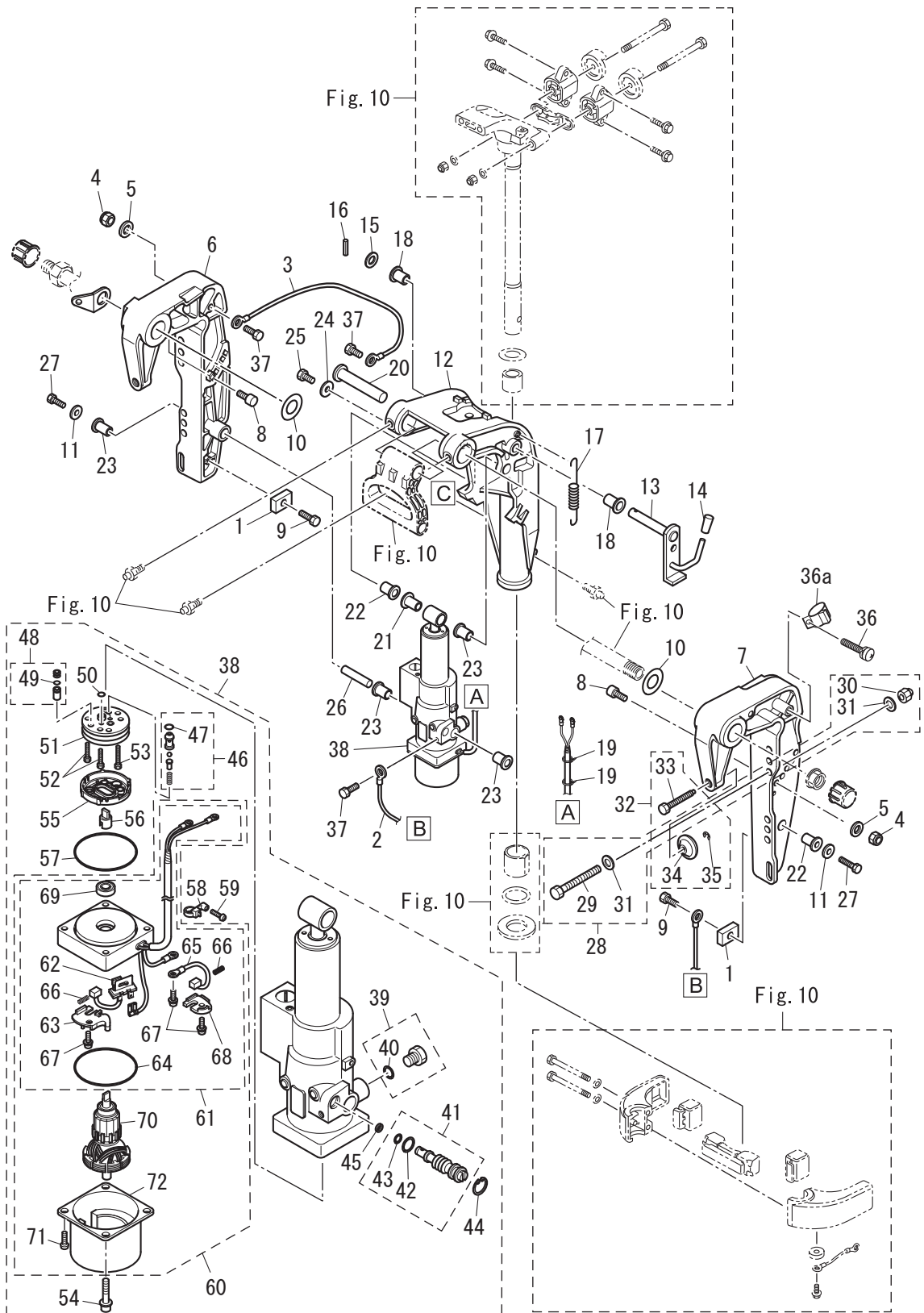
Fig. 11 BRACKET (PT) ブラケット (PT)
