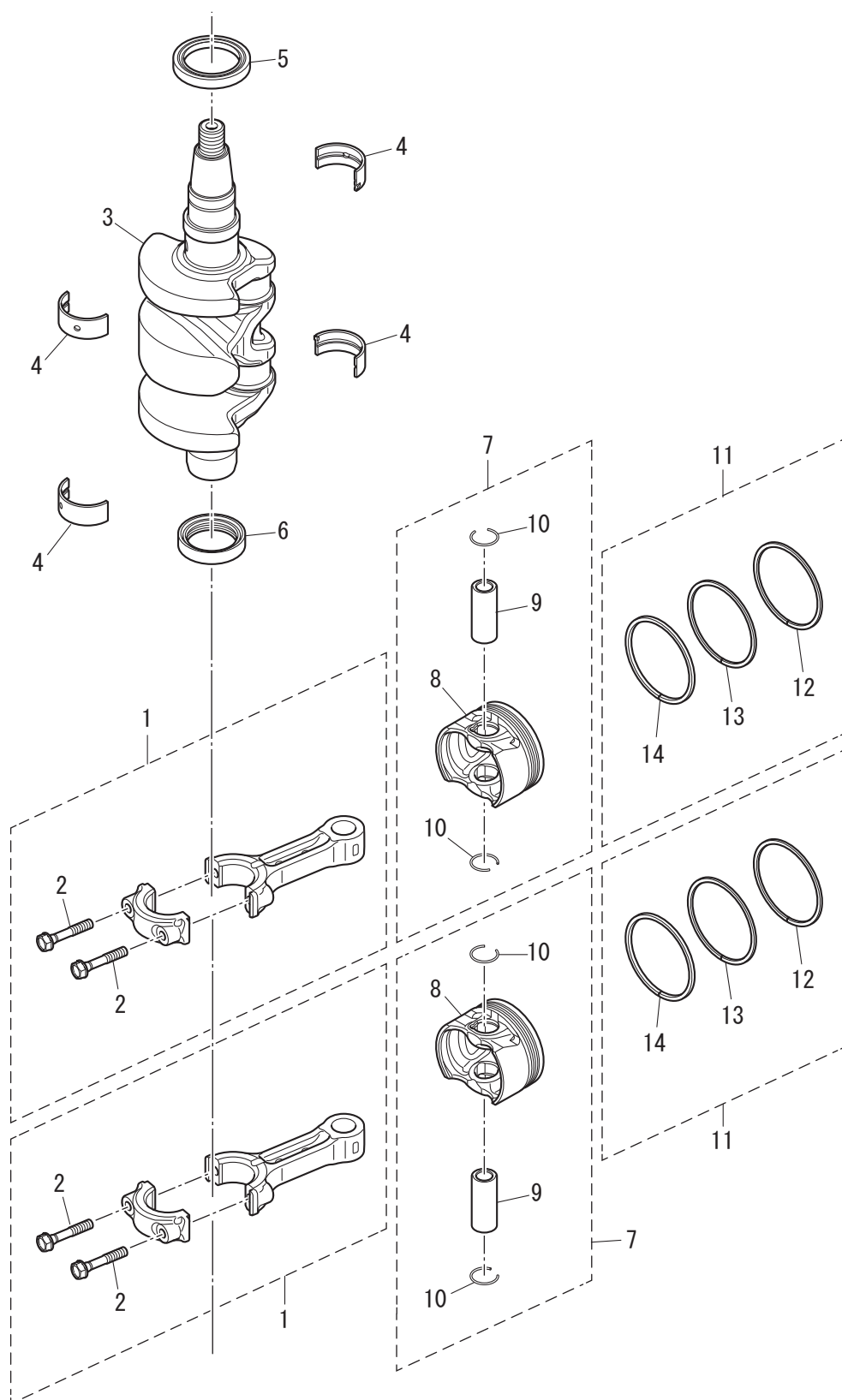
Fig. 2 PISTON · CRANK SHAFT ピストン · クランクシャフト
