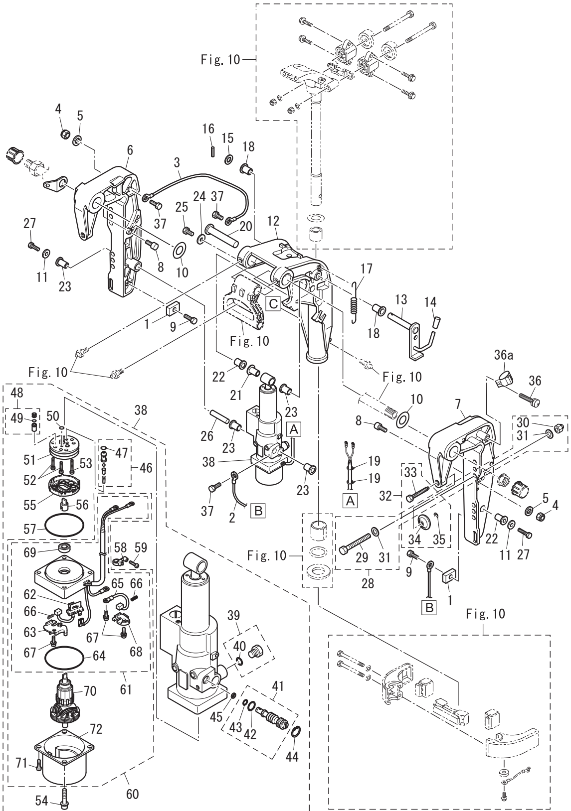
BRACKET (PT) ブラケット (PT)
