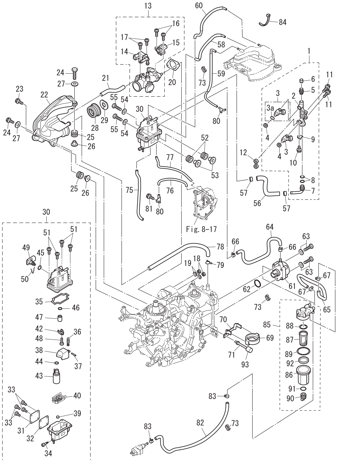
Fig. 5 FUEL PUMP フュエルポンプ
