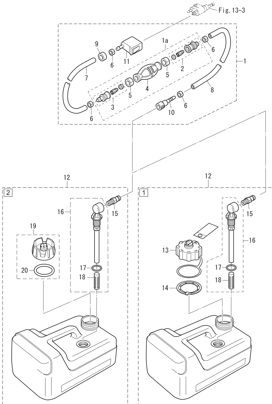
Fig. 16 FUEL TANK フュエルタンク
