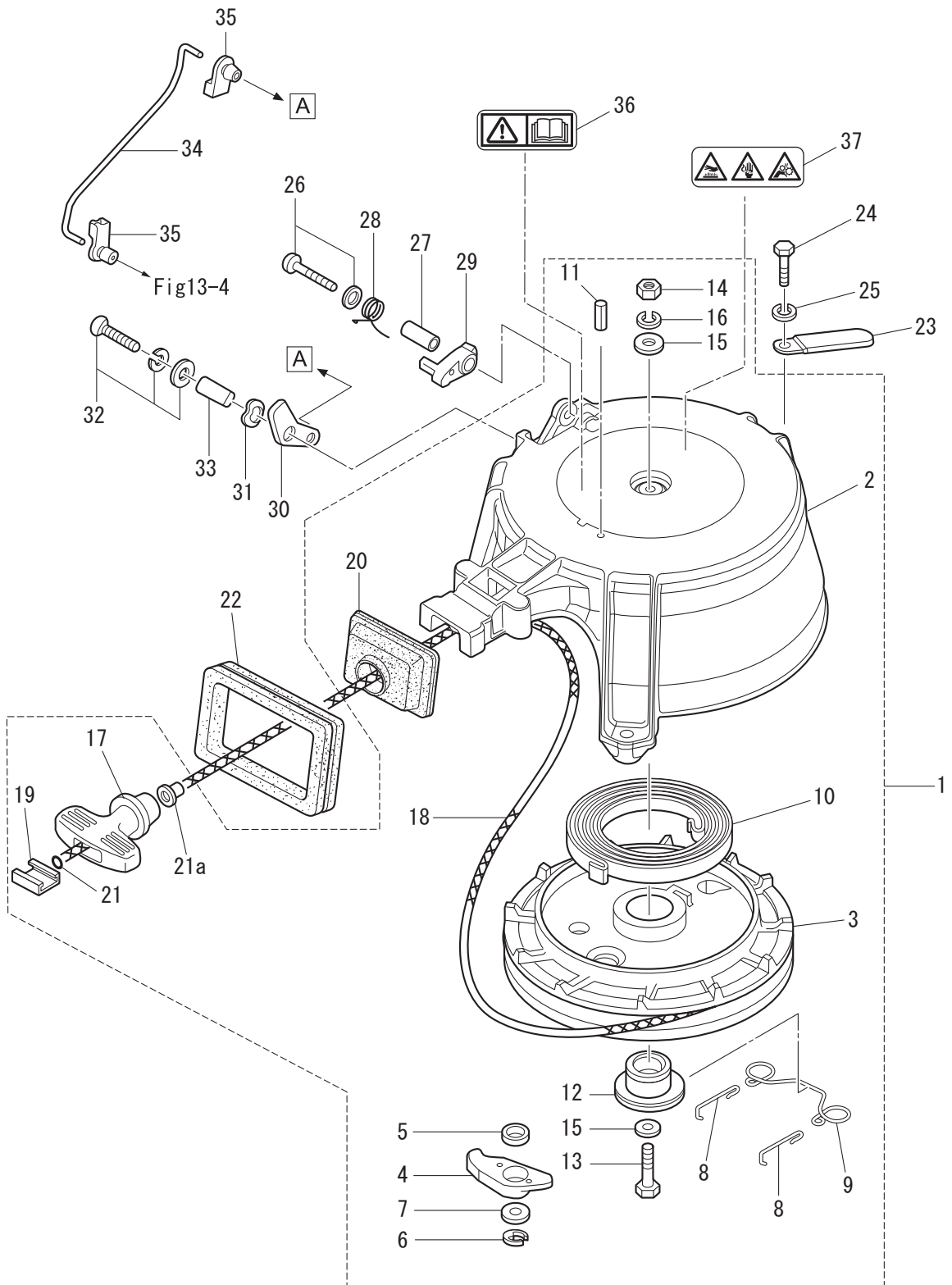
Fig. 5 RECOIL STARTER リコイルスタータ
