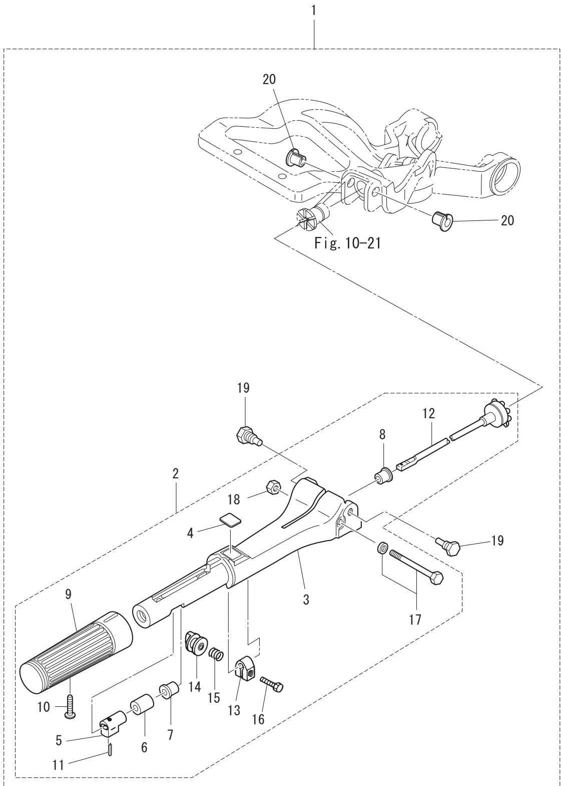
Fig. 11 TILLER HANDLE ティラハンドル
