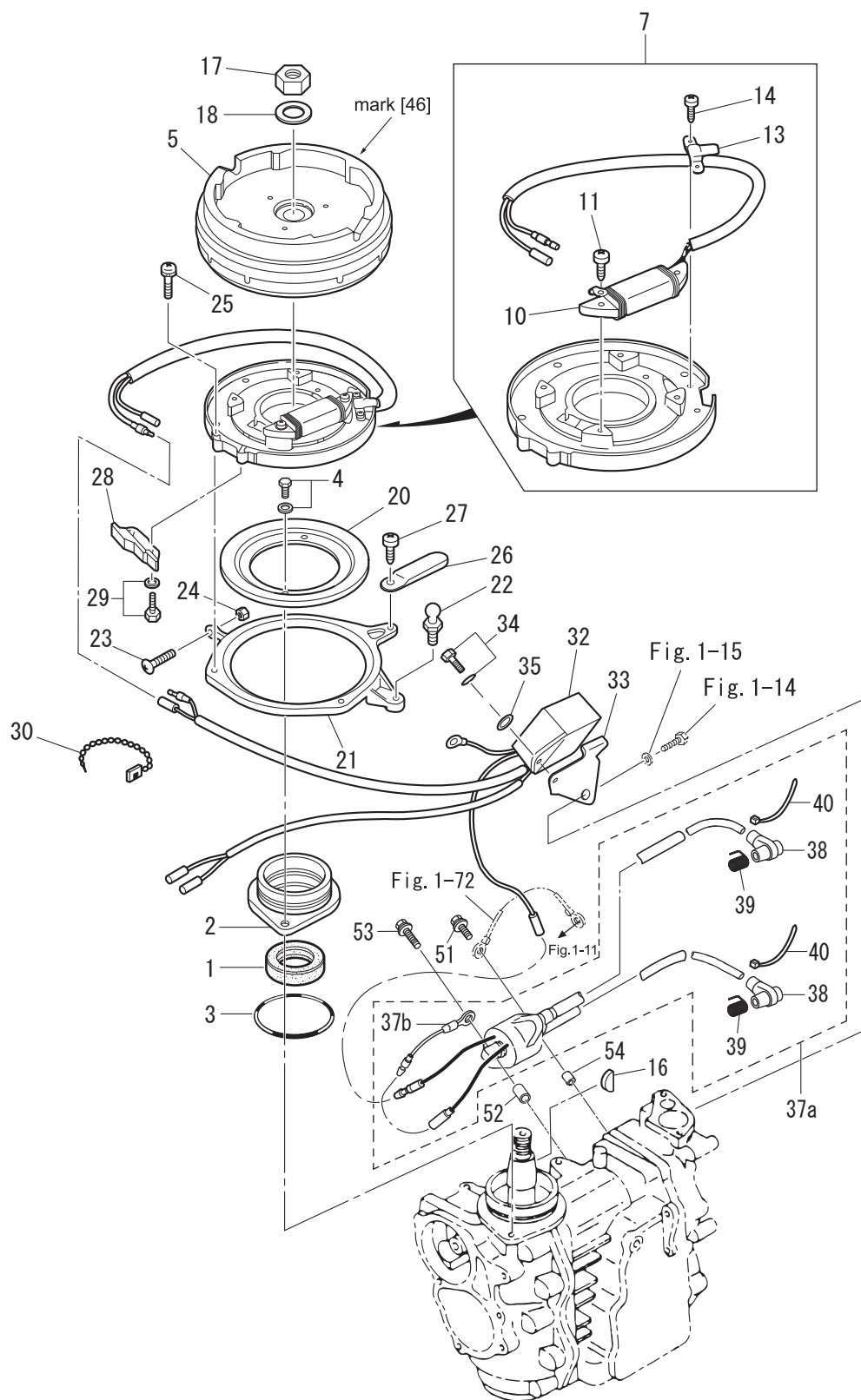
Fig. 6 MAGNETO · ELECTRIC PARTS マグネト · エレクトリックパーツ
