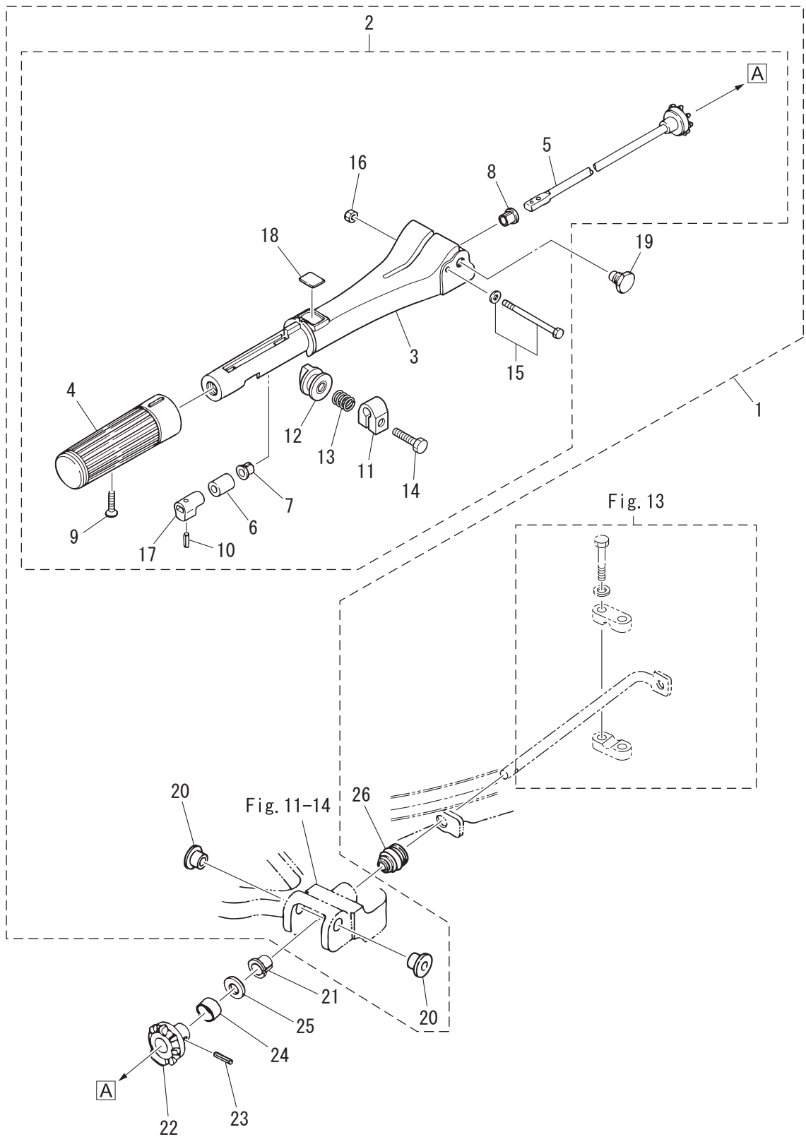
Fig. 12 TILLER HANDLE ティラハンドル
