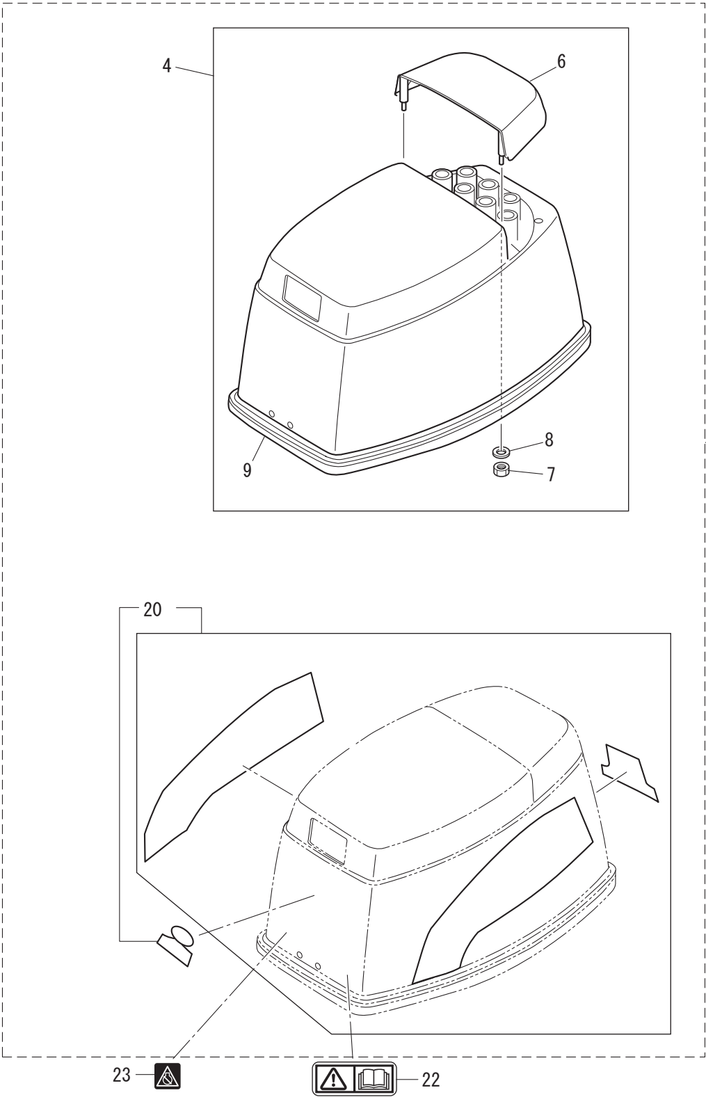
Fig. 24 TOP COWL トップカウル
