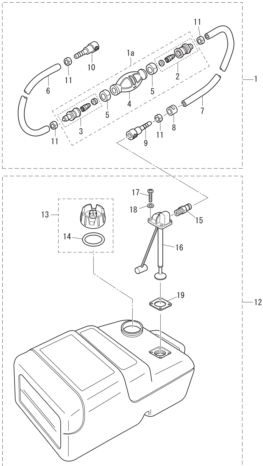
Fig. 25 FUEL TANK フュエルタンク
