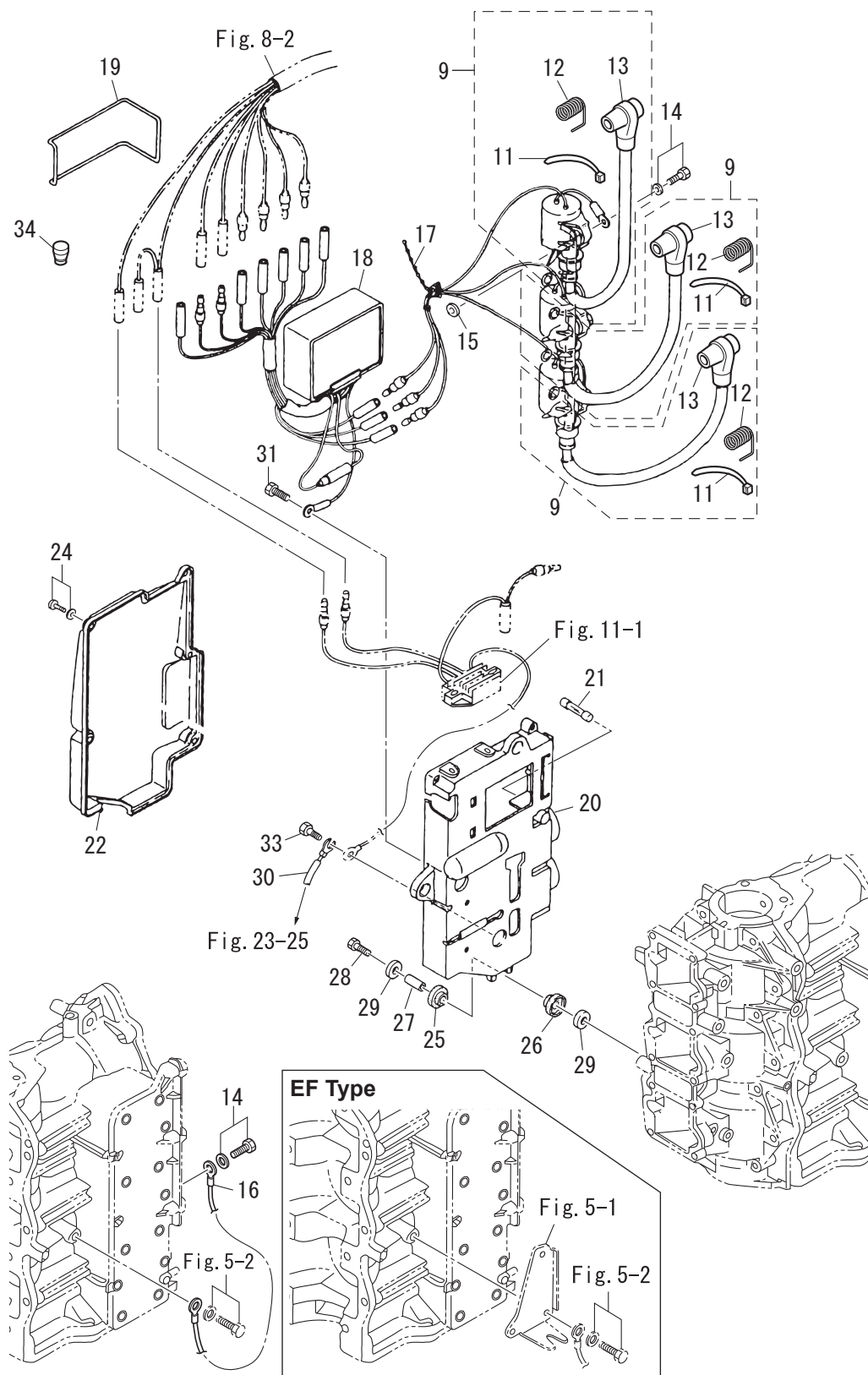
ELECTRIC PARTS (C. D. UNIT) エレクトリックパーツ (C.D. ユニット)
