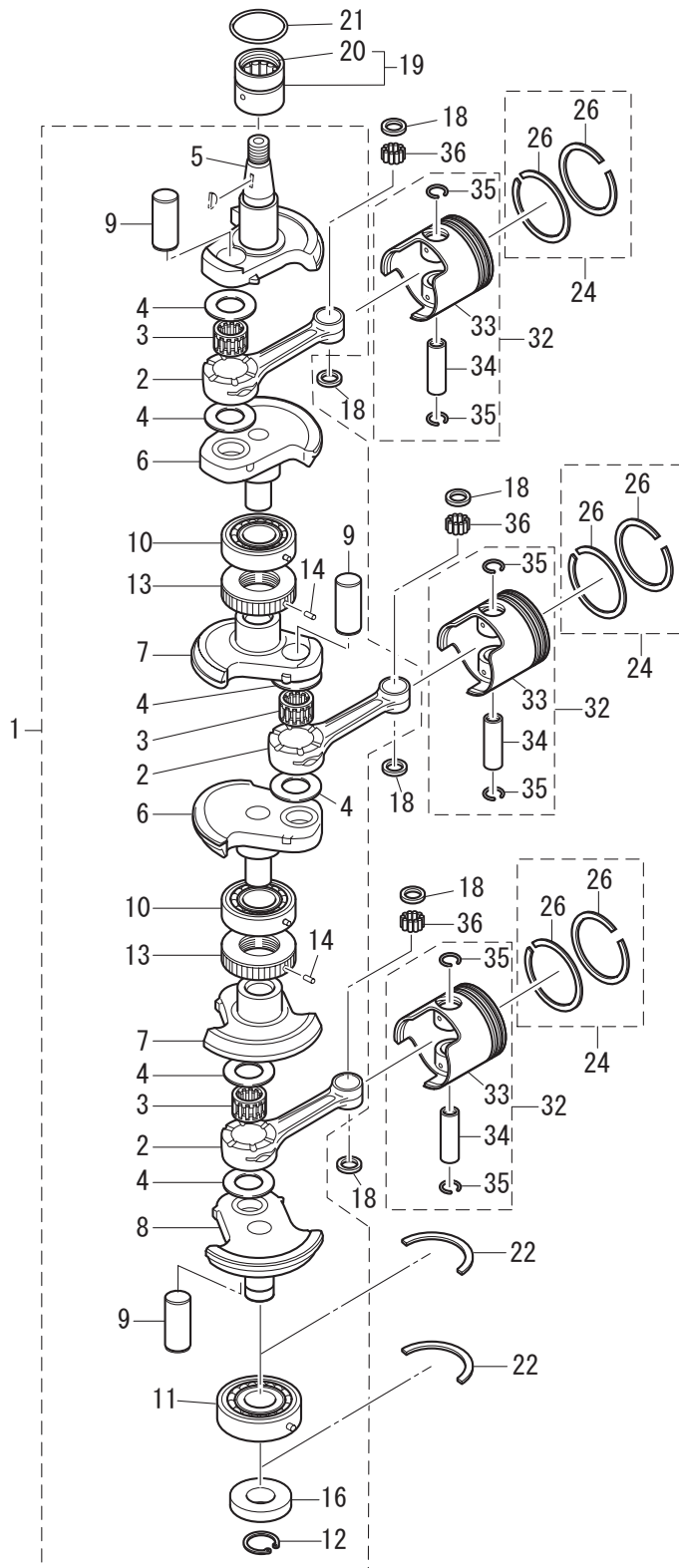
Fig. 2 PISTON · CRANK SHAFT ピストン · クランクシャフト
