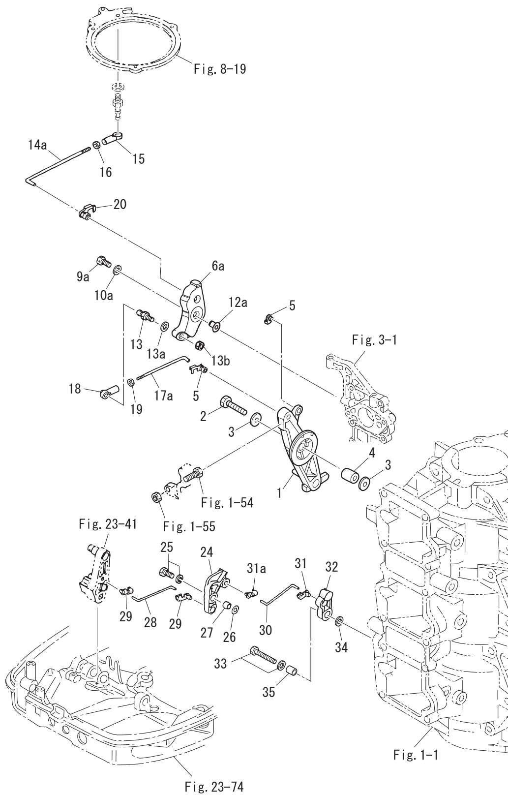
Fig. 6 THROTTLE スロットル
